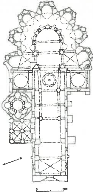
Plan général de l'église (d'après le dossier de présentation à l'UNESCO)
